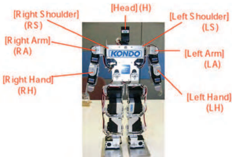
Fig. 2. KHR2-HV
