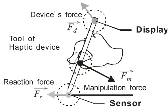
Fig. 11. Sensor & display of SmartTools
