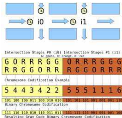
Fig. 2. Chromosome Codification
