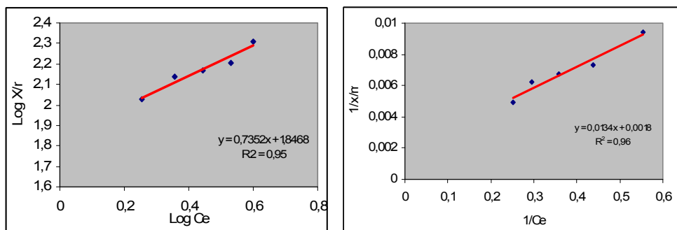
Fig. 5. Freundlich isotherm Figure 6. Langmuir isotherm
