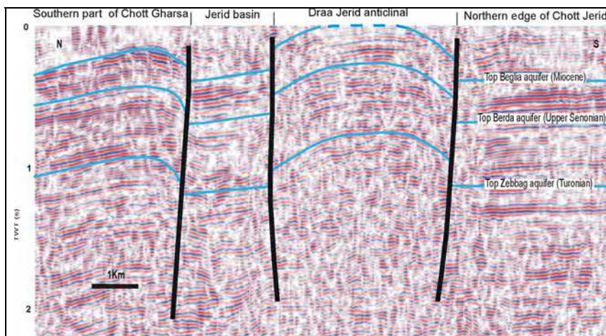
Fig. 11. Seismic section «V» interpretation.
