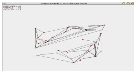
Fig. 15. Generation 300, graph 10028.
