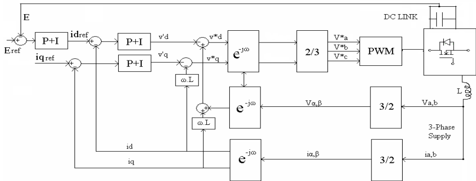
Fig. 11. DQ Control lock diagram.
