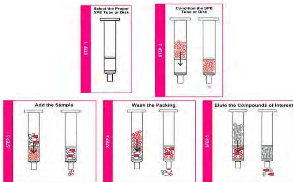
Fig. 3. SPE procedure steps (Supelco, 1998).
