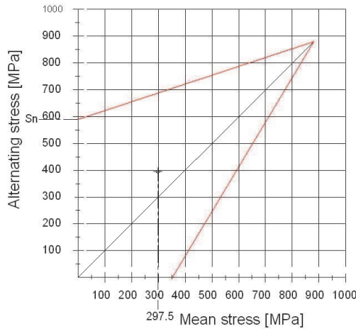
Fig. 4. Goodman’s diagram. Ti6Al4V
