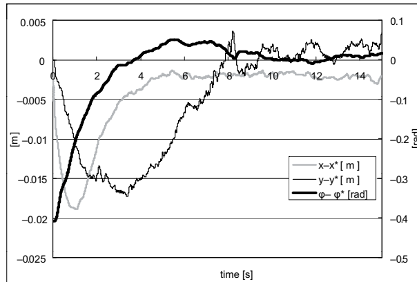
Fig. 9. Position error trajectories
