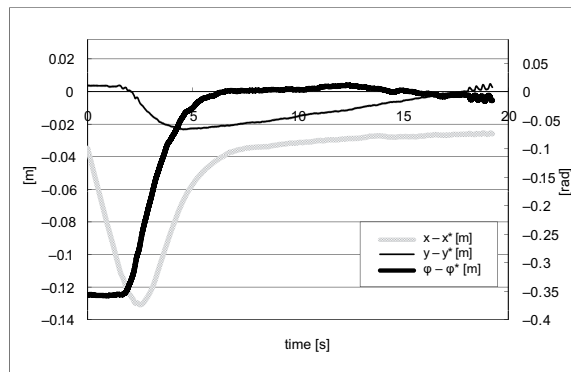
Fig. 11. Position error trajectories
