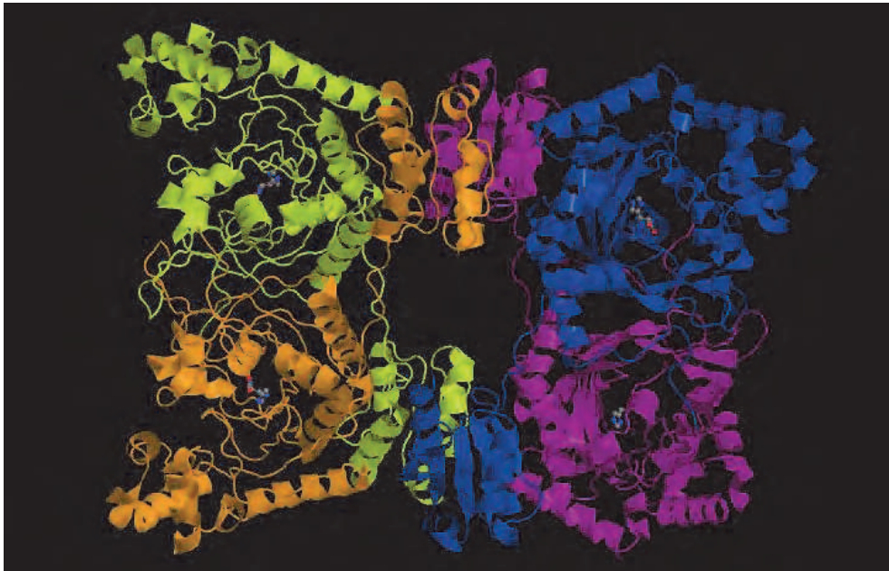
Fig. 2. Histidyl tRNA Ligase tetramer (Aberg et al., 1997).
