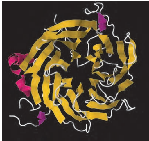
Fig. 4. The NURD complex (Lejon et al., 2011b).
