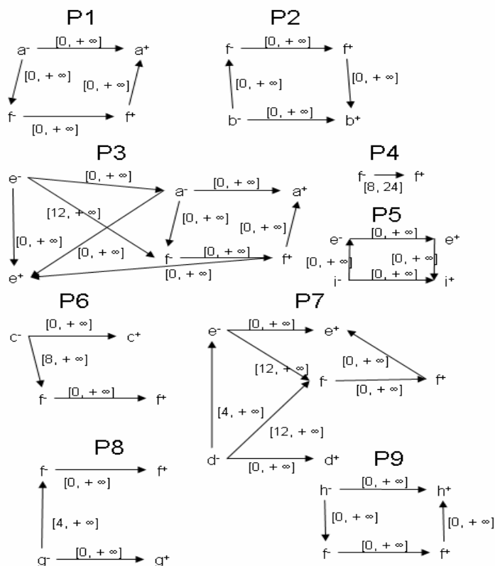
Fig. 13. Plans for CSAR mission
