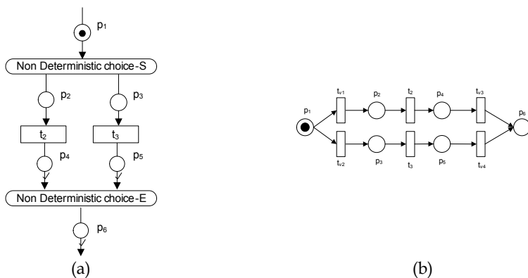
Fig. 5. Non deterministic choice
