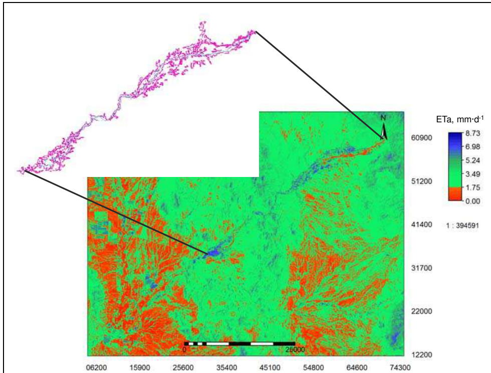
Fig. 8. ETa values for DOY143
