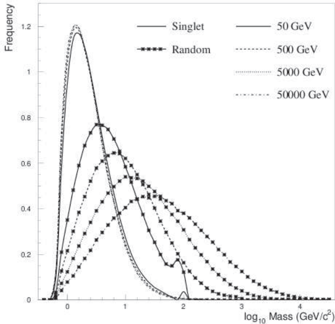
Fig. 6. Preconfinement
