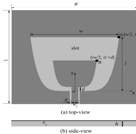
Figure 19. Binomial slot antennas.
