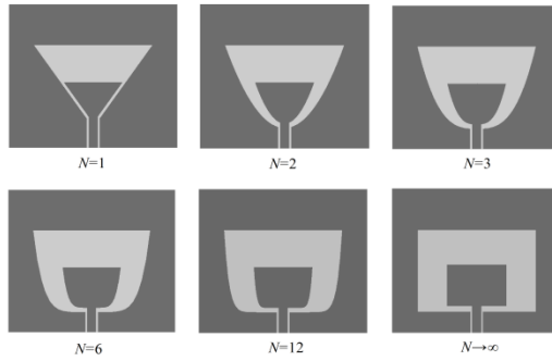
Figure 20. Various binomial slot antennas.
