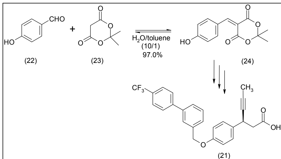
Fig. 5. AMG 837 (21) synthesis.
