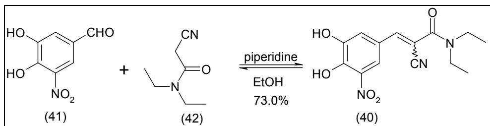
Fig. 10. Entacapone (40) synthesis.
