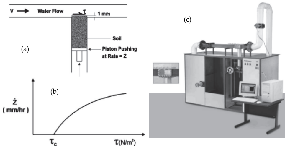
Fig. 12. Erosion Function Apparatus –EFA– (Briaud et al., 2001)
