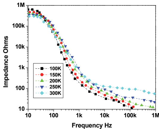
Fig. 15a. Impedance spectra of ITO/PEDOT:PSS/Alq3/Al.
