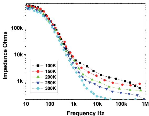
Fig. 15b. Impedance spectra of ITO/PEDOT:PSS/Alq3/LiF/Al.
