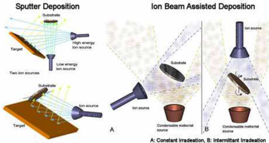
Fig. n.4. Deposition Configuration
