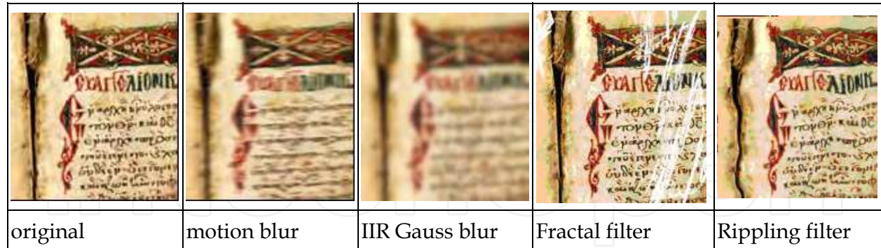
Fig. 27. Blur filters
