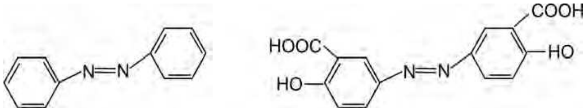
Azobenzene
