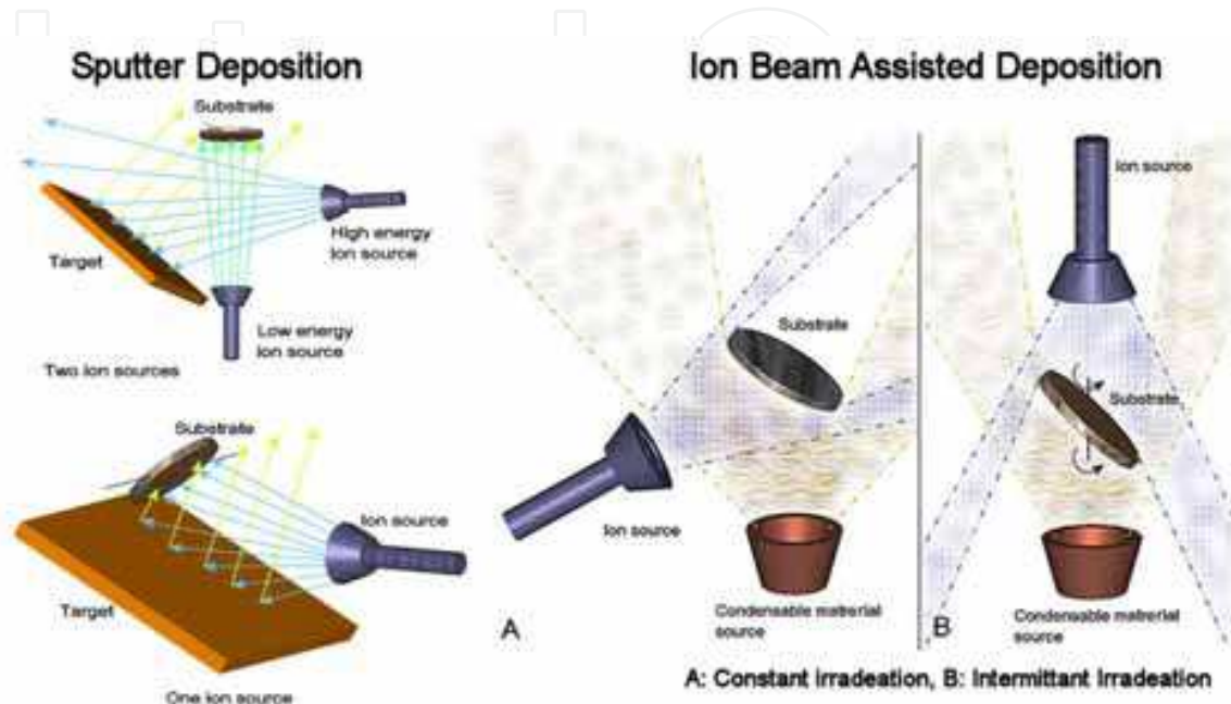
Fig. n.4. Deposition Configuration
